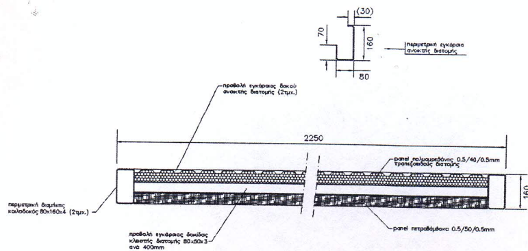
ΤΟΜΗ ΟΡΟΦΗΣ
