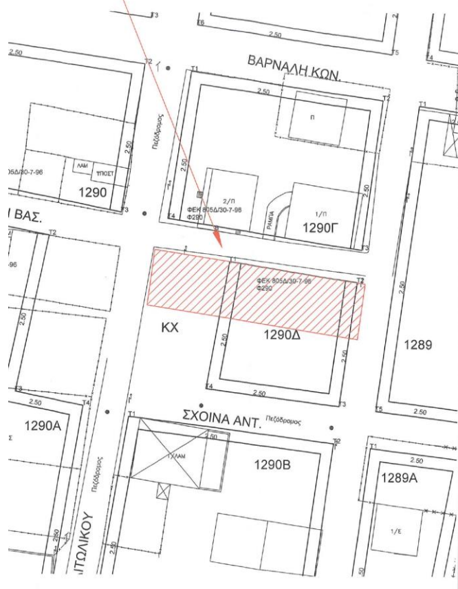
ΑΠΟΣΠΑΣΜΑ ΔΙΑΓΡΑΜΜΑΤΟΣ Ο.Τ. Κλίμακα 1/500 ΘΕΣΗ ΟΙΚΟΠΕΔΟΥ
