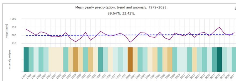
Εικόνα 7: Ετήσια Μεταβολή Βροχοπτώσεων στην περιοχή της Λάρισας έτη 1979 – 2021
