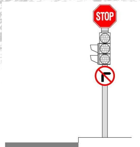
Σχήμα 2. Τοποθέτηση πινακίδων στον ιστό του σηματοδότη
