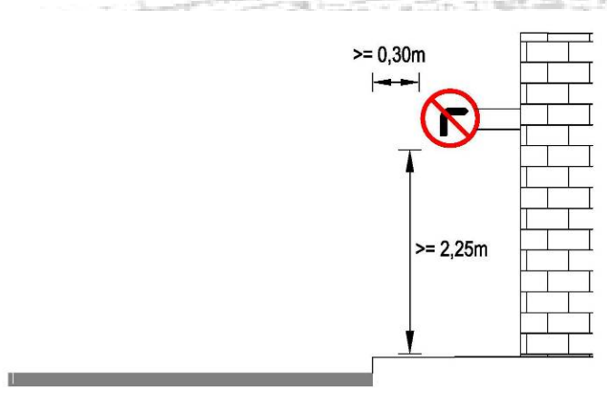
Σχήμα 3. Στήριξη πινακίδας σε τοίχο σε αστικές περιοχές
