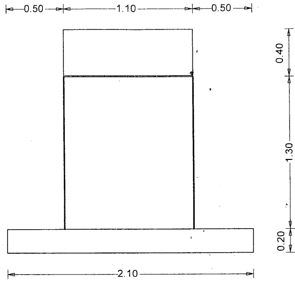
ΕΜΠΡΟΣ ΟΨΗ
