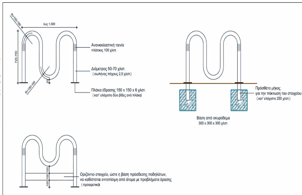
Σχήμα 0-6 Σωληνοειδή μεταλλικά στηρίγματα μορφής M για την πρόσδεση ποδηλάτων
