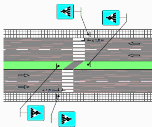
β. Σε οδούς διαχωρισμένης επιφάνειας κυκλοφορίας
