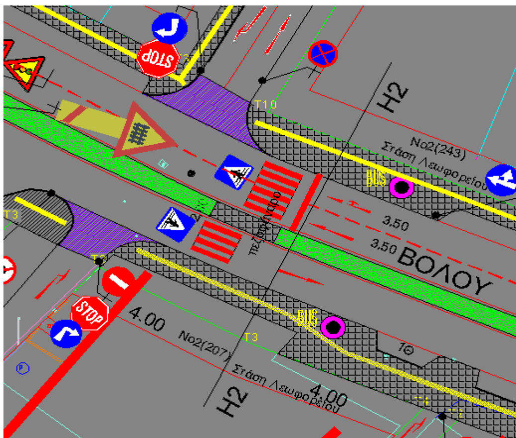
ΤΥΠΙΚΗ ΔΙΑΤΟΜΗ Η2 ΒΟΛΟΥ (ΜΠΑΣΔΕΚΗ/ΑΝΩΝΥΜΟΣ)
