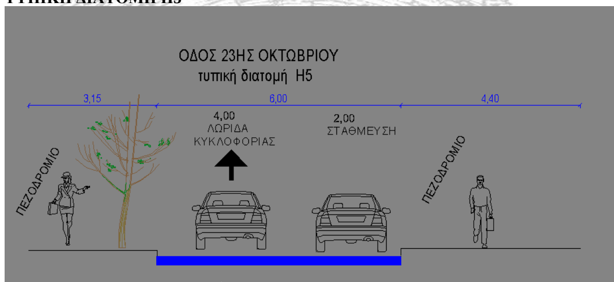
ΤΥΠΙΚΗ ΔΙΑΤΟΜΗ Η5
