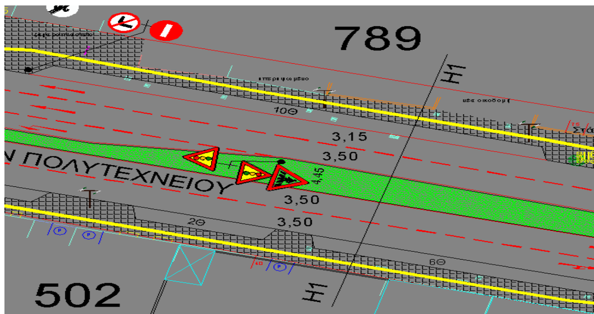
ΤΥΠΙΚΗ ΔΙΑΤΟΜΗ Η1 ΗΡ. ΠΟΛΥΤΕΧΝΕΙΟΥ (ΚΑΡΔΙΤΣΗΣ/ΠΑΠΑΝΑΣΤΑΣΙΟΥ – ΑΒΕΡΩΦ)
