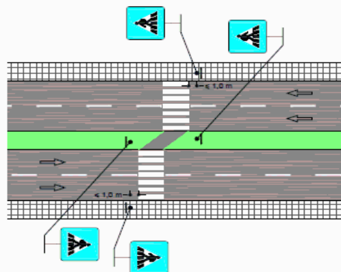
β. Σε οδούς διαχωρισμένης επιφάνειας κυκλοφορίας
