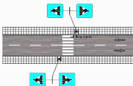
α. Σε οδούς ενιαίας επιφάνειας κυκλοφορίας
